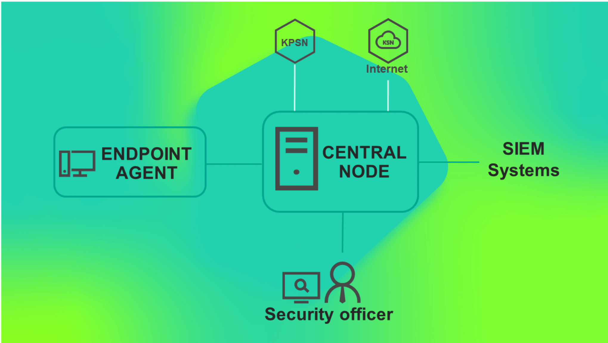
Схема работы приложения при развертывании функциональности KEDR без компонента Sandbox
