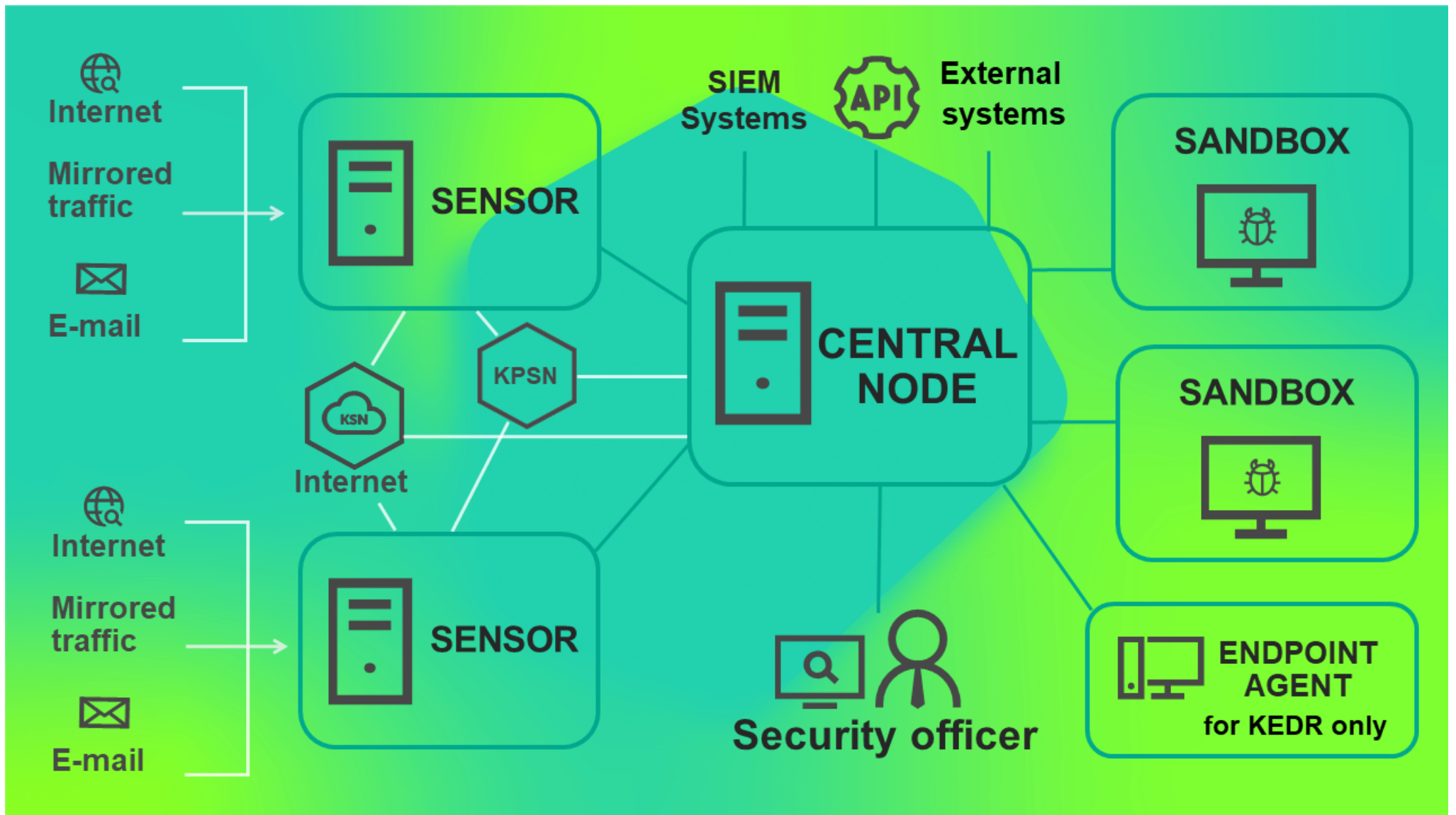
Схема работы приложения при развертывании на четыре и более сервера
